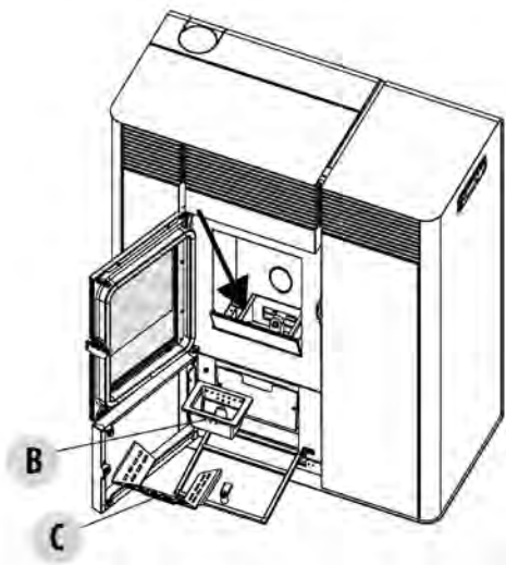
Fig. 20 - Entnahme Aschenlade
