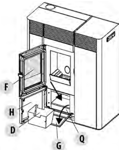
Fig. 21 - Entnahme Brennschale
