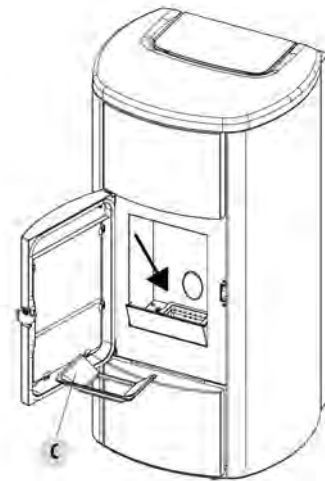
Fig. 19 - Entnahme Brennschale
