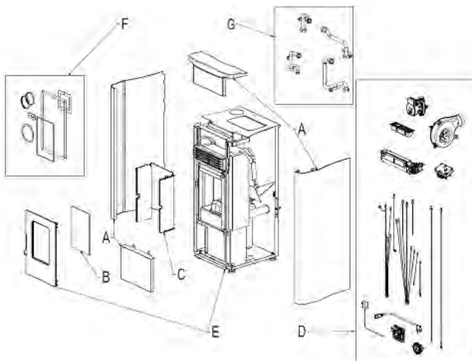
Explosionszeichnung
